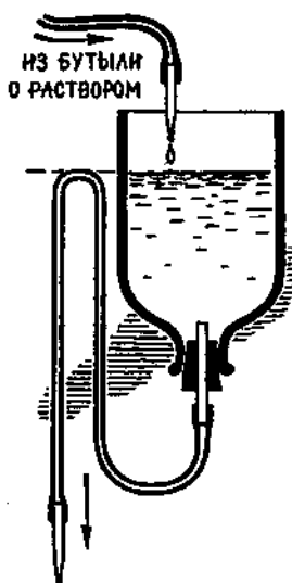
Как сделать сифон для смачивания корней отдельными порциями раствора.
