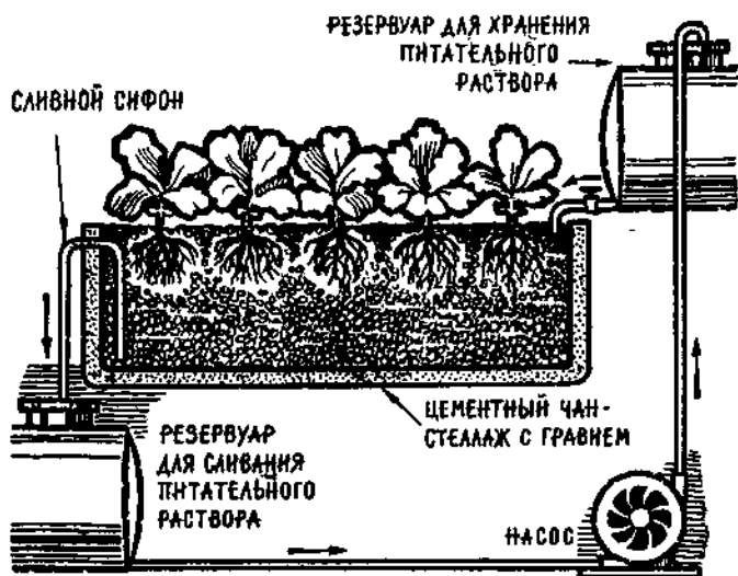
Схема гравийной гидропонии.
