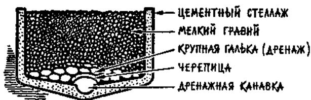
Поперечный разрез гравийной гидропонники.
